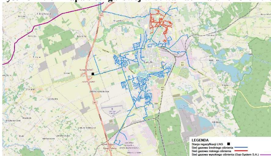
Rysunek 4.2.2 Mapa sieci gazowej w Suwałkach na dzień 31.12.2021 r.
