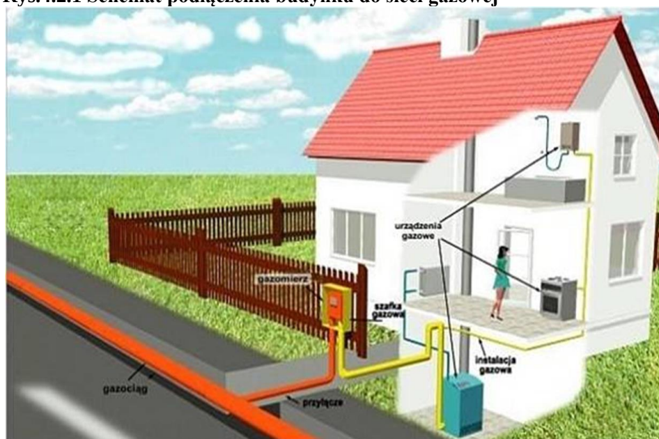
Rys.4.2.1 Schemat podłączenia budynku do sieci gazowej
